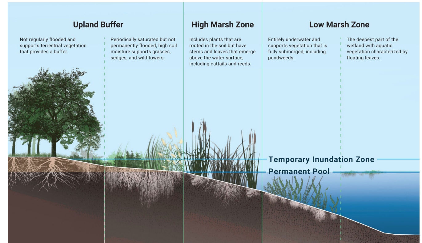
Figure 10-8. Wetland zones
