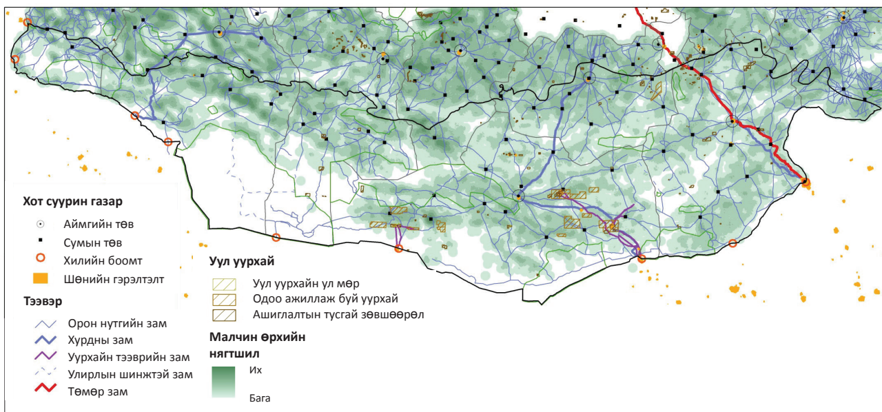
Зураг 11: Нөлөөллийн индекс.
