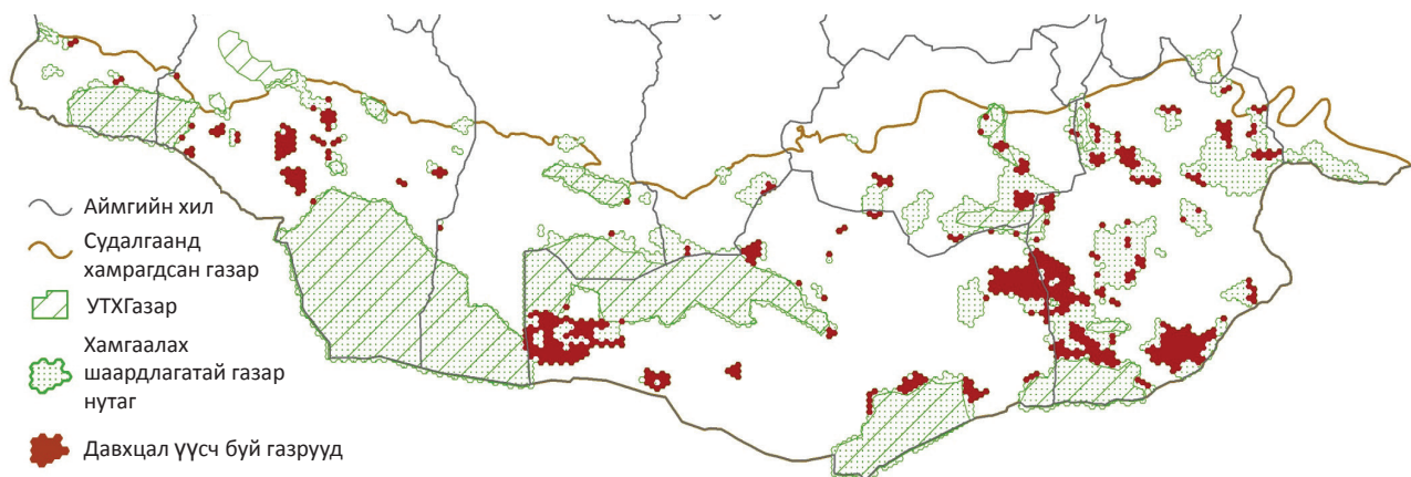
Зураг 17: Хамгаалах шаардлагатай газар нутгууд ба ашигт малтмалын тусгай зөвшөөрлийн талбайтай давхцалтай газрууд.
