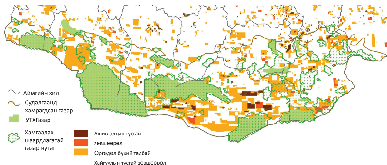
Зураг 16: Хамгаалах шаардлагатай газар нутгийн эхний хувилбар болон ашигт малтмалын тусгай зөвшөөрөл олгосон газрууд.
