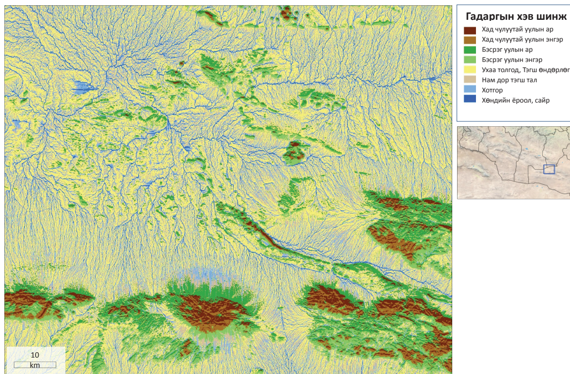
Зураг 8: Газрын гадаргын хэв шинж. Өндрийн тоон загварын (DEM) топографын гурван индексийг ангилах замаар гаргасан. Үүний үр дүнд говь, цөлийн бүсэд гадаргын хэлбэрийн 8 хэв шинжийг тодорхойлж зураглал хийсэн. Бид үүнийг 1) түгээмэл экосистемийг тогтоох ба 2) сонгосон төлөөлөл зүйлийн хувьд тэдний амьдрах орчны тархацыг загварчилахад ашигласан.
