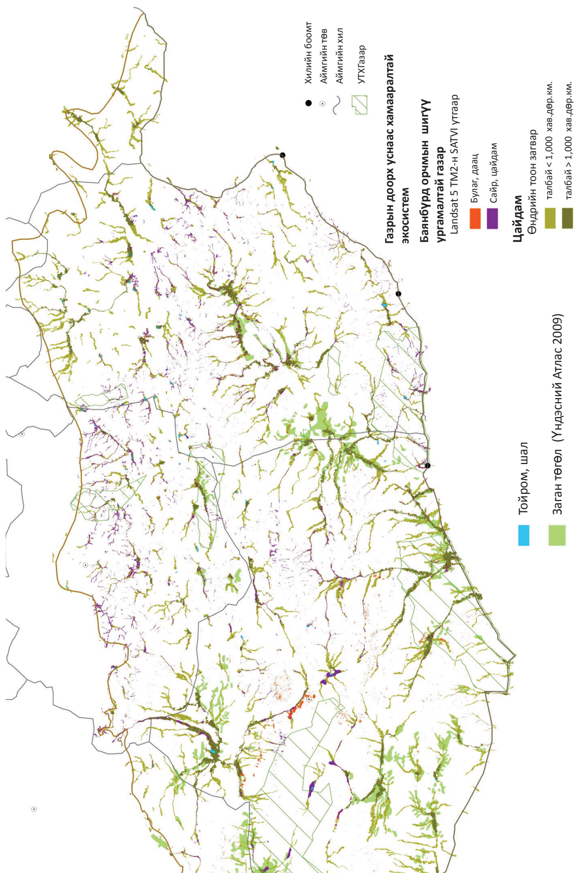
Зураг 276: Газрын доорх уснаас хамааралтай экосистемийн хэв шинж: Судалгаанд хамрагдсан бүс нутгийн дорнод хэсэг.
