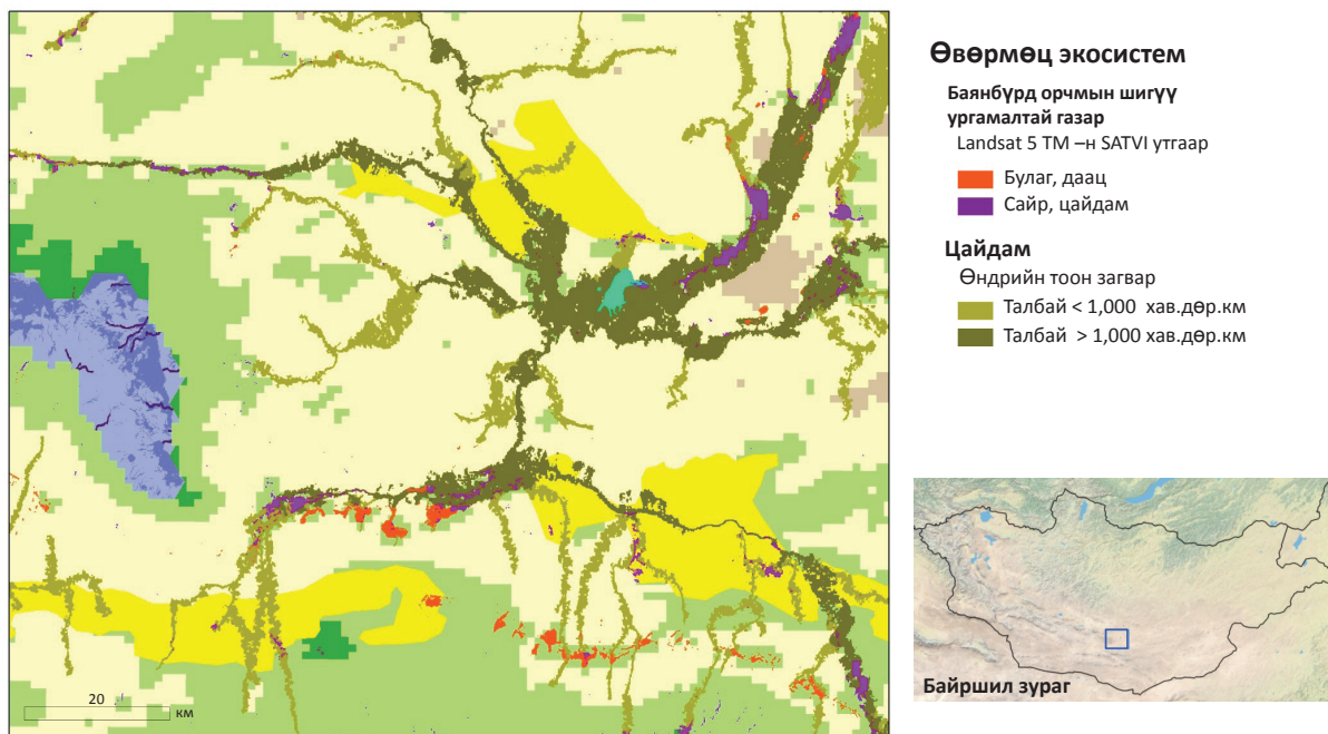
Зураг 7в: Газрын экосистемийн ангилал — Өвөрмөц экосистемийг тодруулж харуулав.
