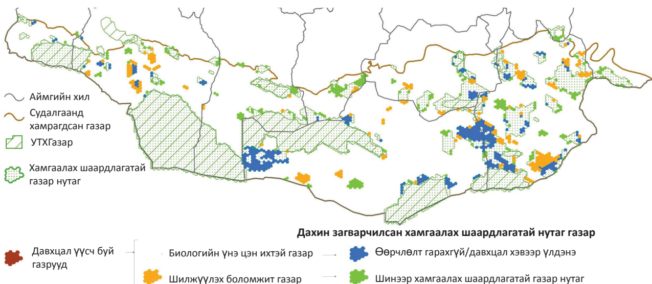
Зураг 19: Хамгаалах шаардлагатай газар нутгууд, ашигт малтмалын тусгай зөвшөөрлийн давхцалыг багасгах зорилгоор дахин загварчилсан байдал.
