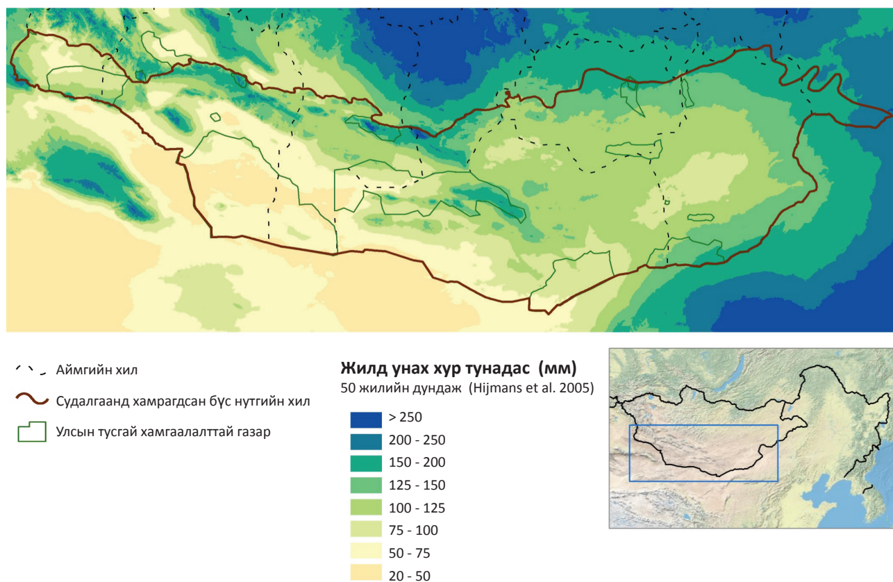
Зураг 2: Судалгаанд хамрагдсан бүс нутаг: Монгол орны өмнийн говь
