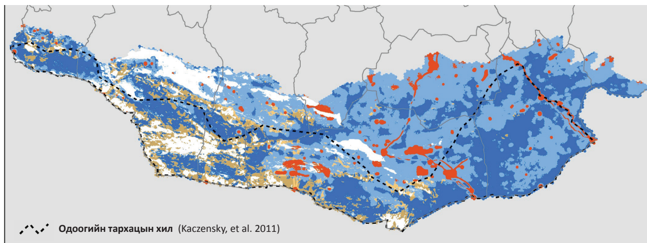
Зураг 15: Хулангийн амьдрах орчны тархацын загвар.
