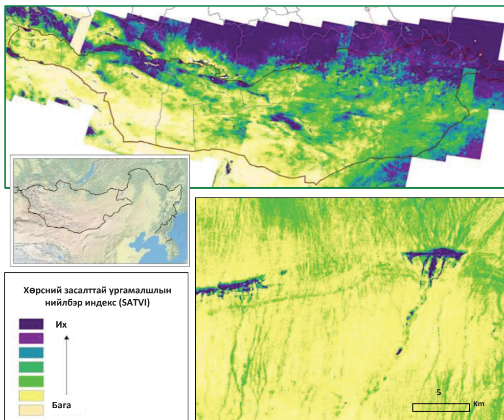
Зураг 1: Өмнөд Монголын Landsat —ын зураг ба булаг шандны эргэн тойрон дах ургамалжилт нягтшил ихтэй байгааг харуулсан хөрсний засалттай ургамалшлын нийлбэр индекс (SATVI)
