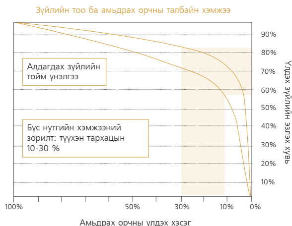
Зураг 9: Зүйл болон амьдрах орчны хамаарлын муруй: Амьдрах орчны талбай болон зүйлийн тоо хэмжээний хоорондын хамаарал. Dobson (1996)-ны загвар
