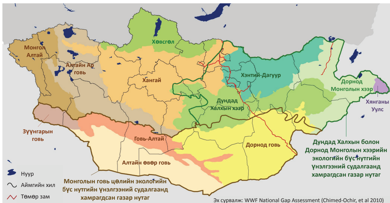
Зураг 1: Монгол орны газрын эко-бүс нутаг.
