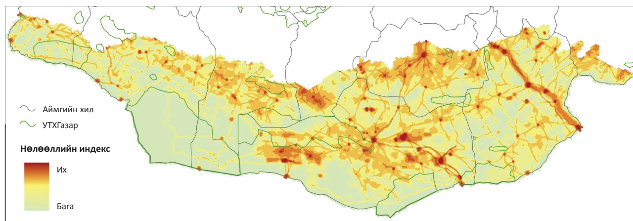
Зураг 11: Нөлөөллийн индекс.
