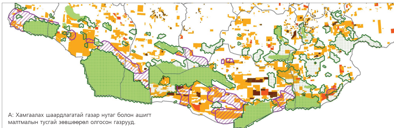
Зураг 22: Хамгаалах шаардлагатай газар нутаг болон ашигт малтмалын тусгай зөвшөөрөл
