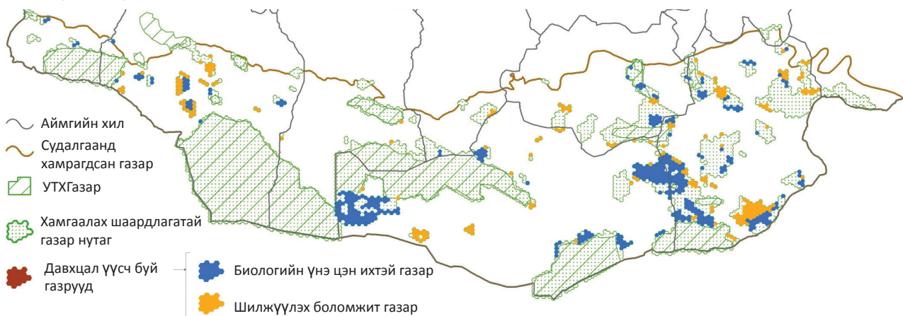
Зураг 18: Хамгаалах шаардлагатай газар нутгууд ба ашигт малтмалын тусгай зөвшөөрөлтэй давхцаж буй зарим газрыг хассан байдал.
