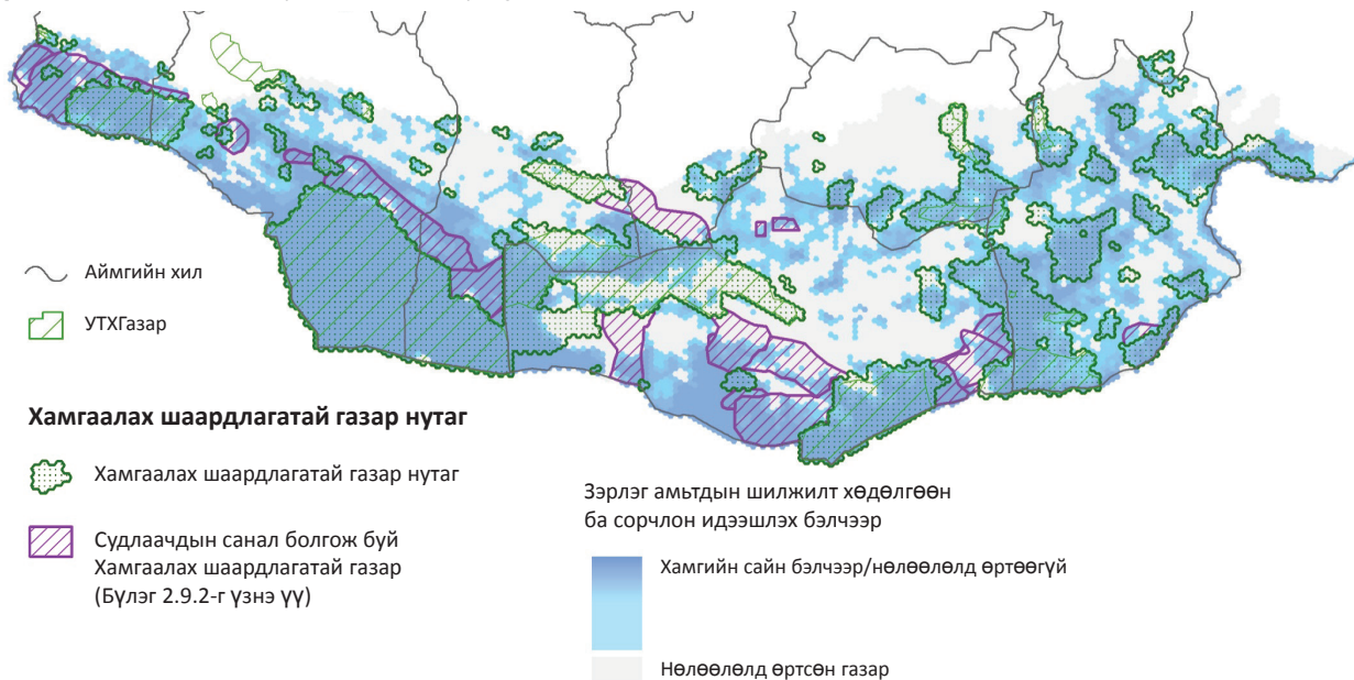
Зураг 21: Хамгаалах шаардлагатай газар нутаг.
